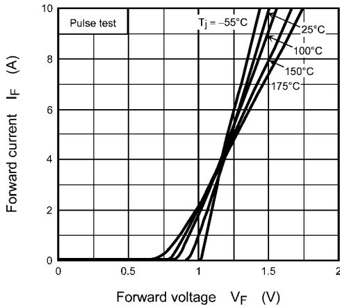
Fig. 9.1 I_F - V_F
