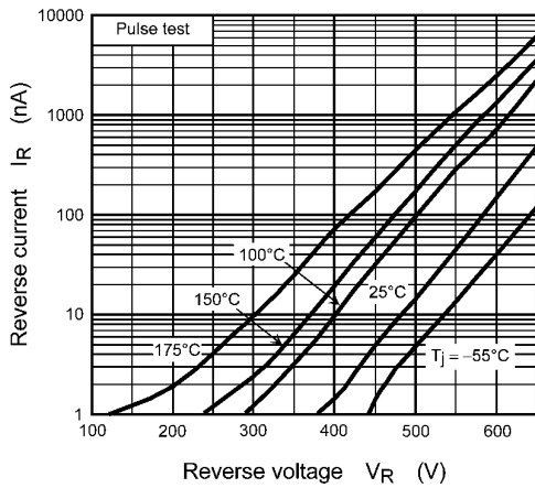
Fig. 9.3 I_R - V_R
