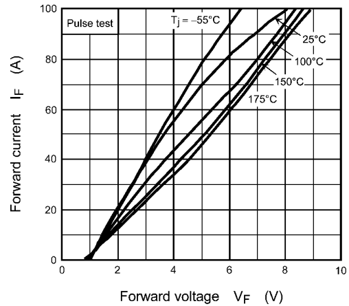
Fig. 9.2 I_F - V_F
